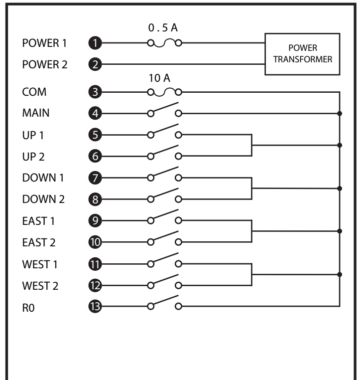
Q404 Wiring diagram
